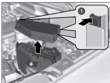
1 Príchytky
